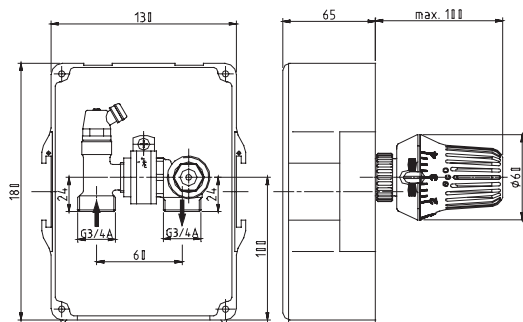
Obrázek 1:RTL-Set s odkrytým ovládáním
