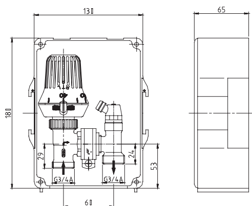
Obrázek 1:RTL-Set s odkrytým ovládáním
